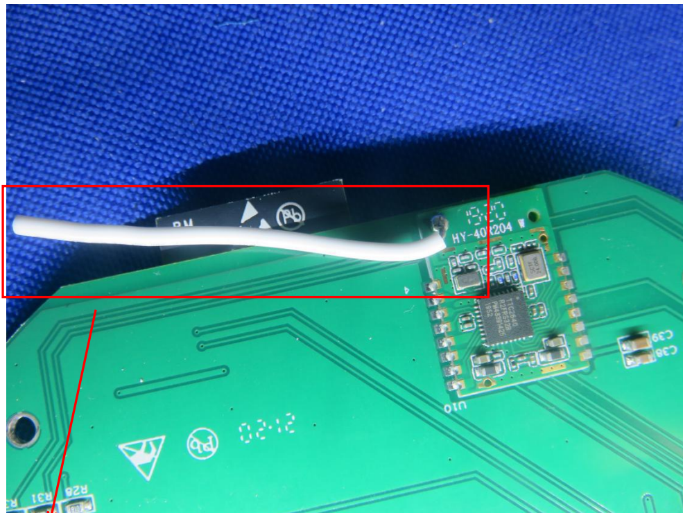
BT ANT
