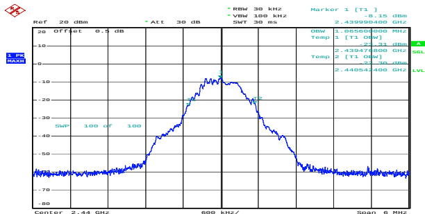
Middle 1.066MHz
