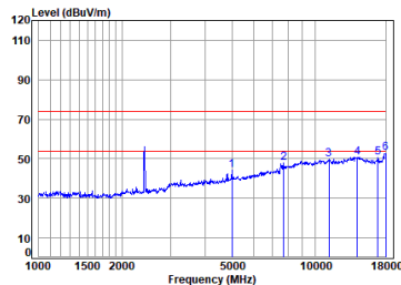
11ax_20M_TX_CH_01_Horizontal
