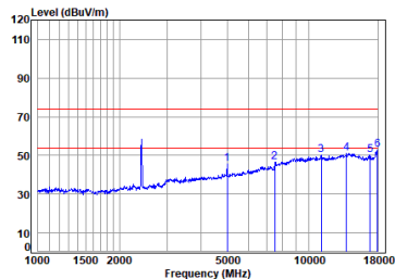
11g_TX_CH_01_Horizontal
