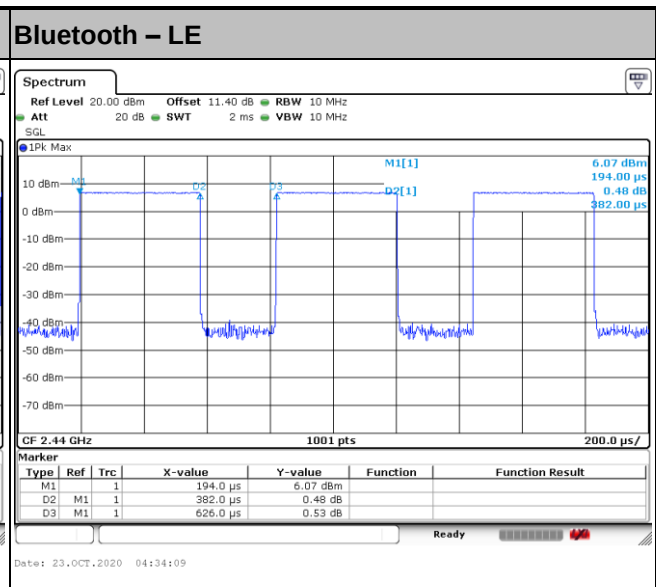
&lt;Ant. 2&gt;
