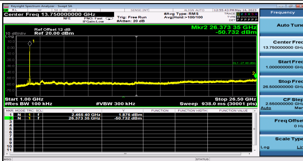
11G_Ant1_2462_1000~26500
