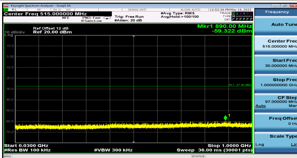
11G_Ant1_2462_30~1000
