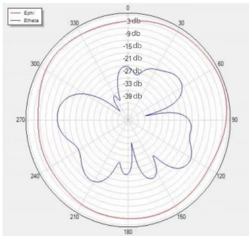
Theta=90 freq=2400MHz
