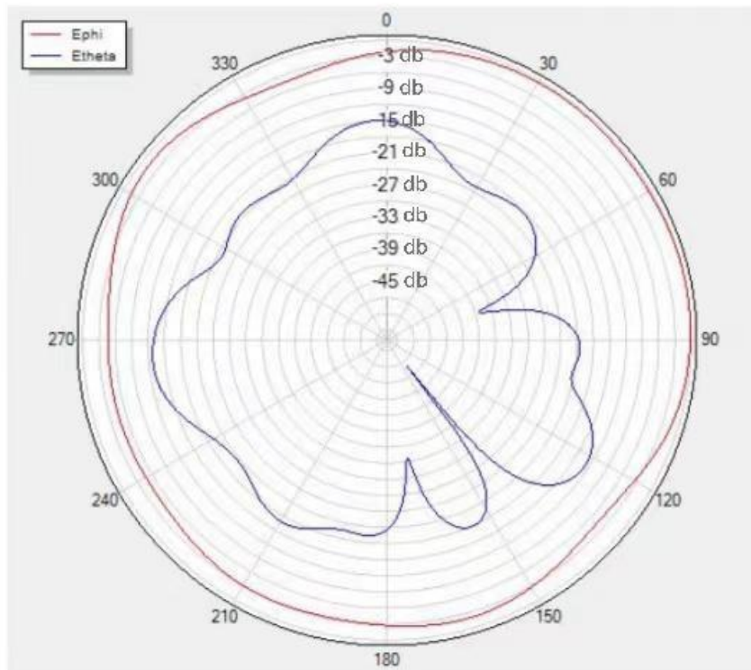
Theta=90 freq=2500MHz
