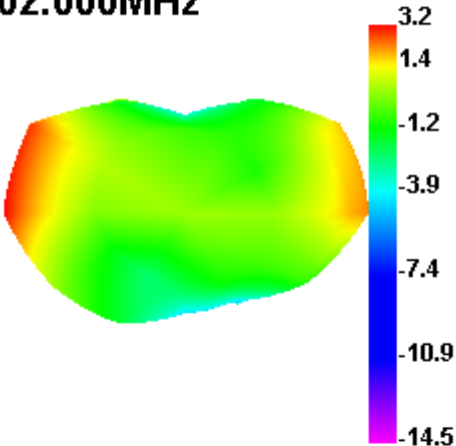
902.000MHz E1
