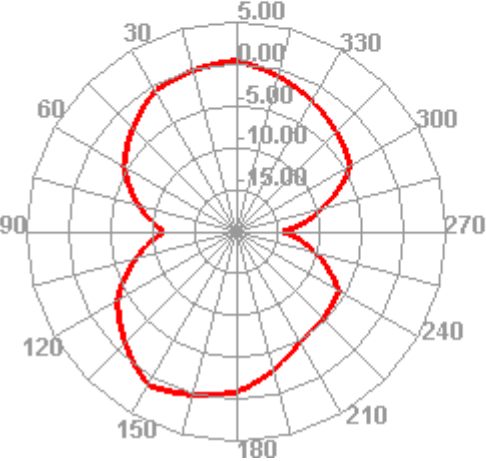
902.000MHz E2
