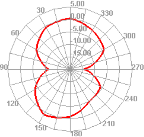
901.000MHz E2
