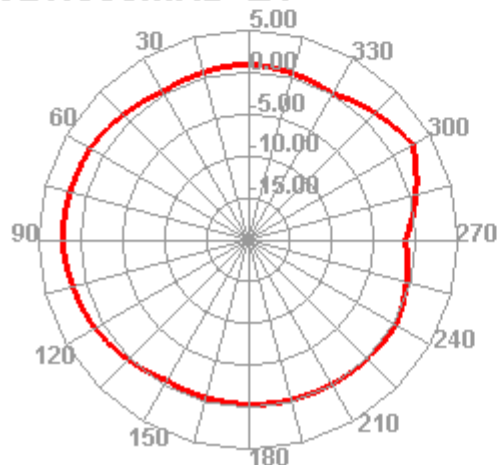
926.000MHz E1
