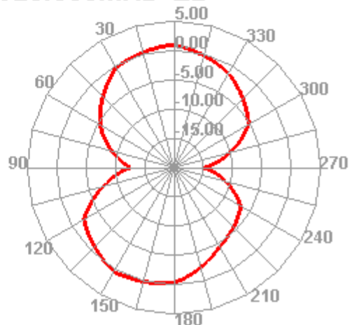
923.000MHz E2
