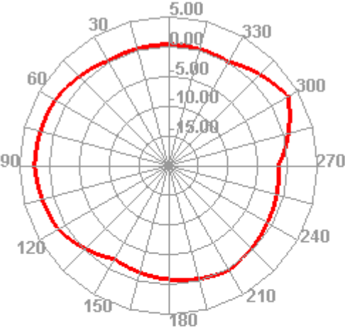
901.000MHz E1
