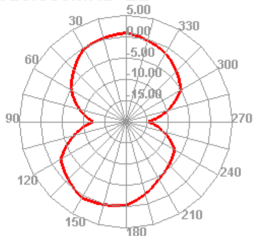
920.000MHz E2
