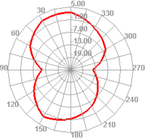
902.000MHz H
