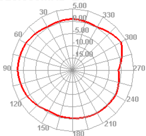
920.000MHz E1
