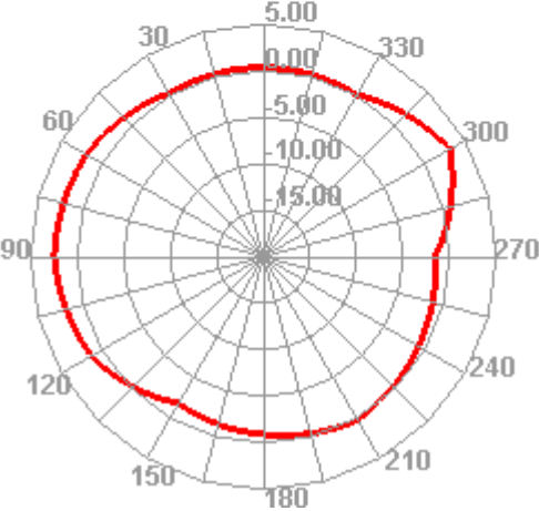
902.000MHz E1
