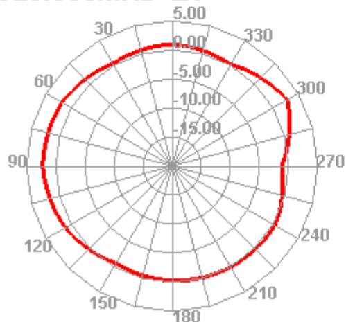
923.000MHz E1
