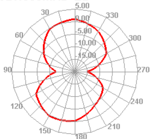
926.000MHz E2
