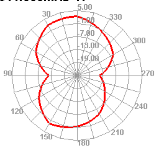
911.000MHz E2
