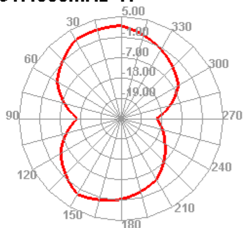
917.000MHz E2
