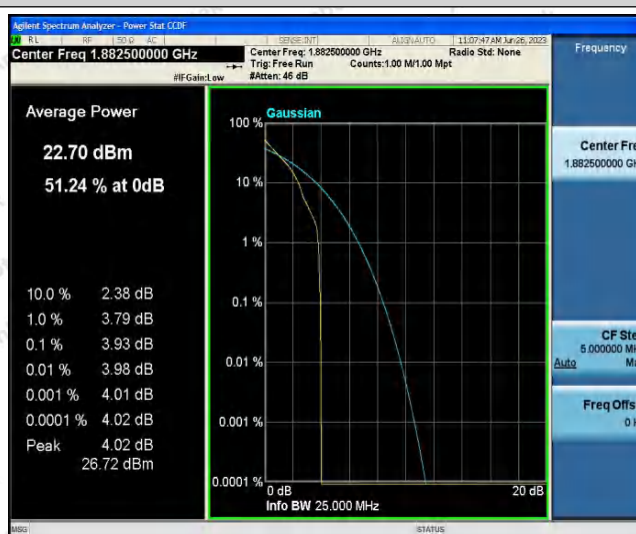
Band25-20MHz-QPSK-26365-100RB#0
