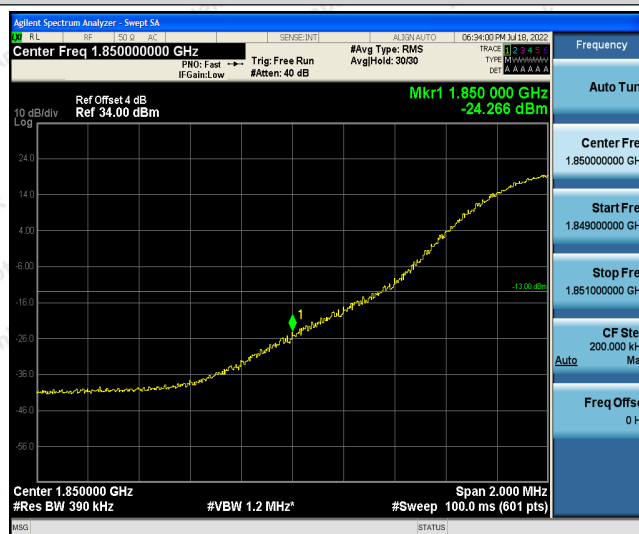
Band2-20MHz-16QAM-18700-1RB#99
