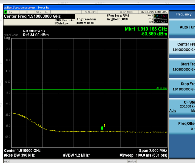
Band2-20MHz-16QAM-19100-1RB#99
