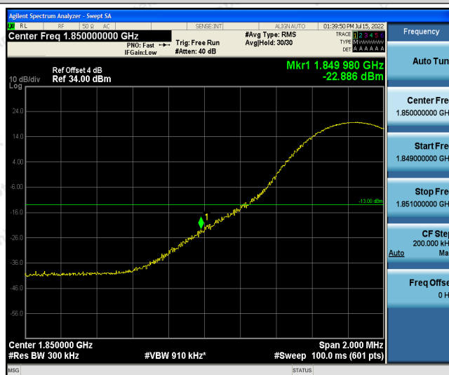
Band2-15MHz-QPSK-18675-1RB#74
