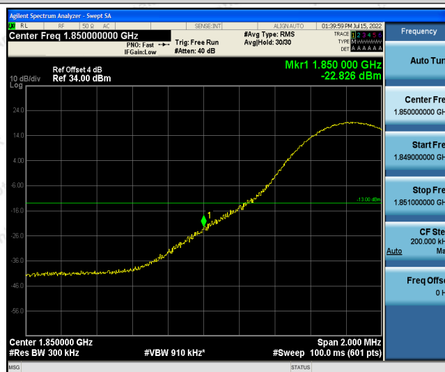
Band2-15MHz-16QAM-18675-1RB#74
