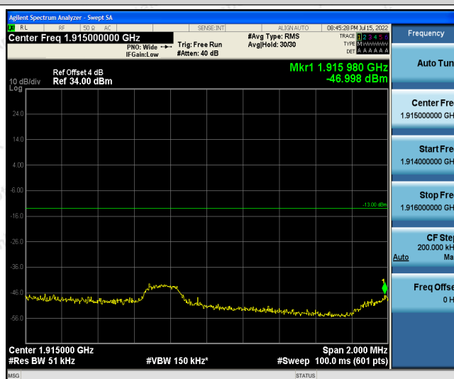
Band25-3MHz-QPSK-26675-1RB#14
