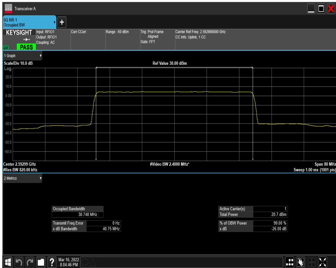
n41 SCS=15kHz CP_QPSK BW=40MHz Channel=518598 RB=216@0
