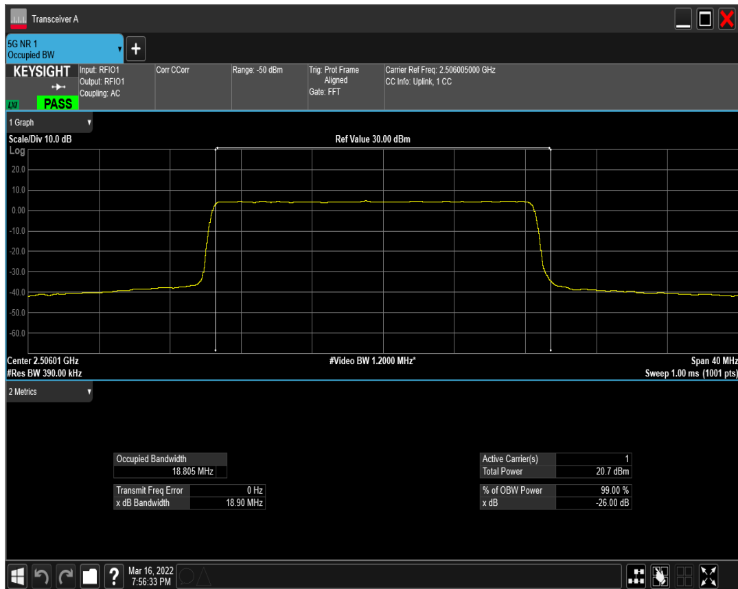
n41 SCS=15kHz CP_QPSK BW=20MHz Channel=501201 RB=106@0
