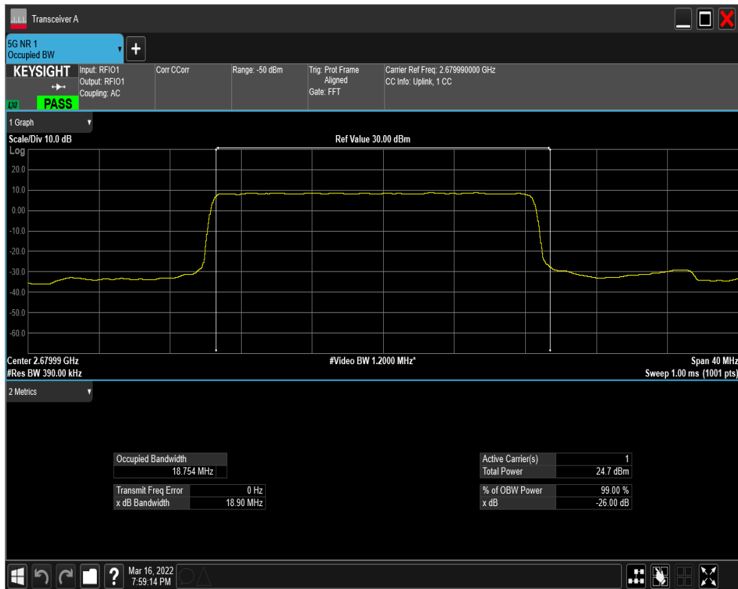
n41 SCS=15kHz DFT_QPSK BW=20MHz Channel=535998 RB=100@0
