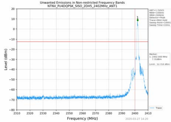
Pi/4DQPSK_2402MHz_2DH5_SISO_ANT1
