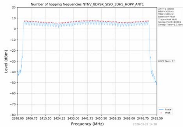
8DPSK_Hopping_3DH5_SISO_ANT1
