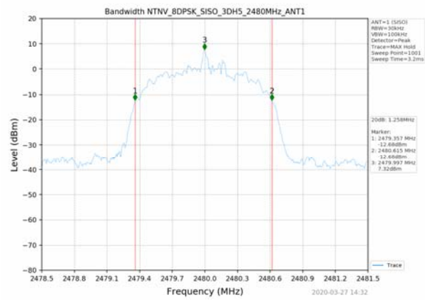
8DPSK_2480MHz_3DH5_SISO_ANT1
