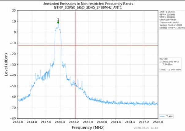
8DPSK_2480MHz_3DH5_SISO_ANT1
