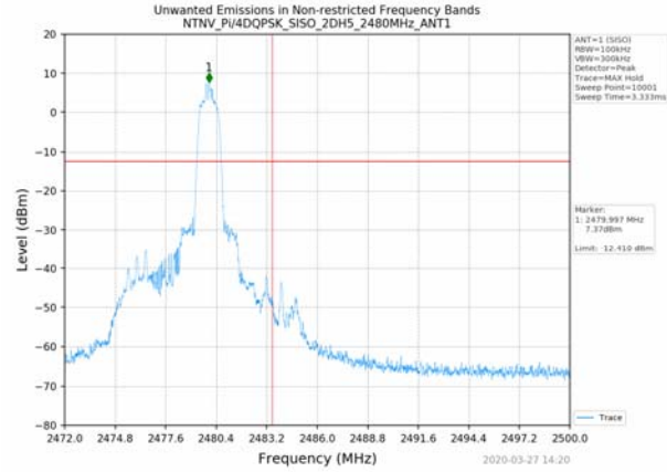
Pi/4DQPSK_2480MHz_2DH5_SISO_ANT1
