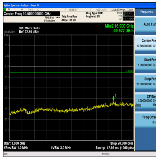
Band2-5MHz-QPSK-18625-25RB#0-Range2:1000~20000MHz
