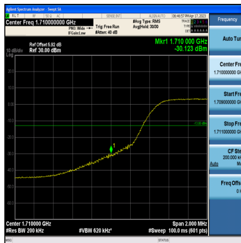
Band66-10MHz-QPSK-132022-50RB#0
