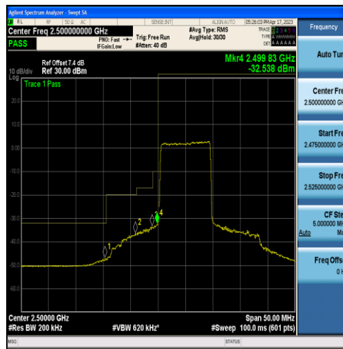
Band7-10MHz-QPSK-20800-50RB#0
