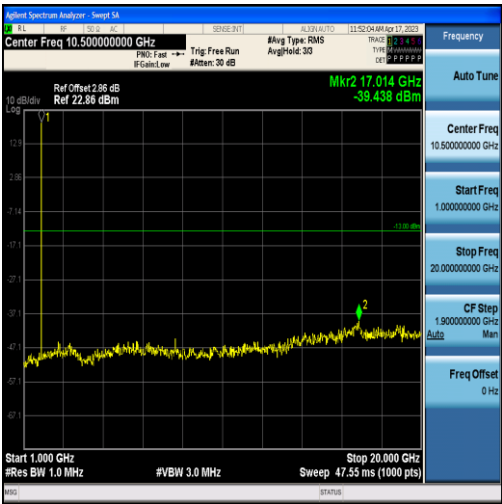
Band2-1.4MHz-QPSK-18607-6RB#0-Range2:1000~20000MHz
