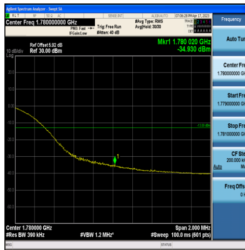
Band66-20MHz-QPSK-132572-100RB#0
