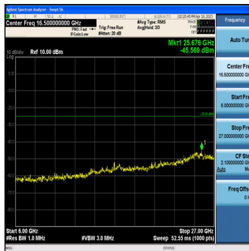
Band7-5MHz-QPSK-20775-25RB#0-Range3:6000~27000MHz
