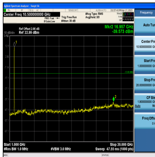
Band4-20MHz-QPSK-20175-100RB#0-Range2:1000~20000MHz
