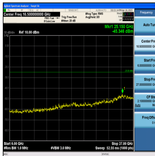
Band7-5MHz-QPSK-21100-25RB#0-Range3:6000~27000MHz
