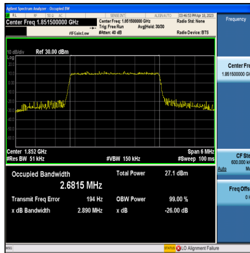
Band2-3MHz-16QAM-18615-15RB#0-2.6815
