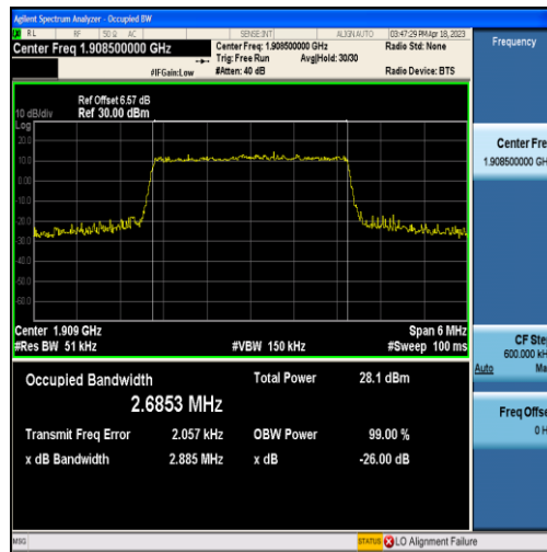
Band2-3MHz-QPSK-19185-15RB#0-2.6853
