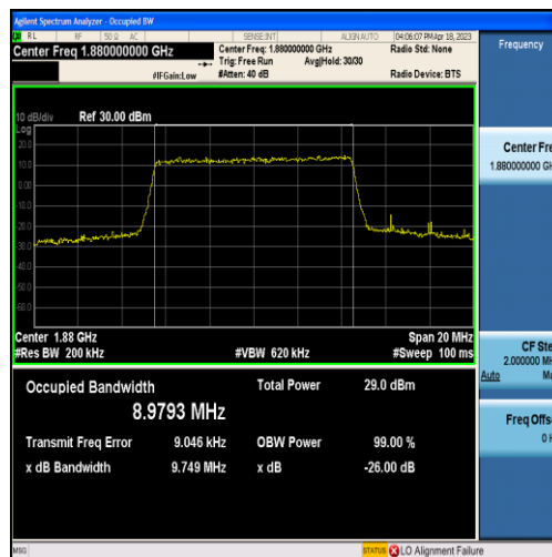
Band2-10MHz-QPSK-18900-50RB#0-8.9793
