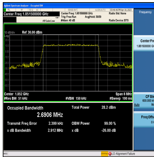
Band2-3MHz-QPSK-18615-15RB#0-2.6906
