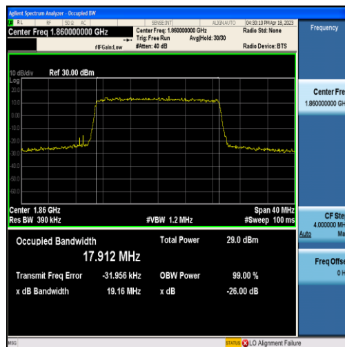
Band2-20MHz-QPSK-18700-100RB#0-17.912
