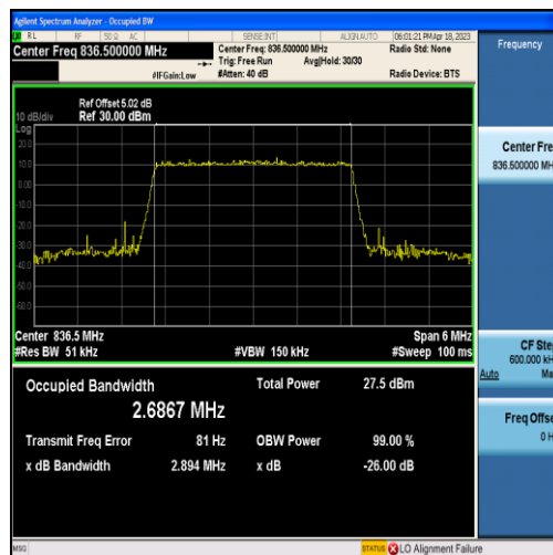
Band5-3MHz-QPSK-20525-15RB#0-2.6867
