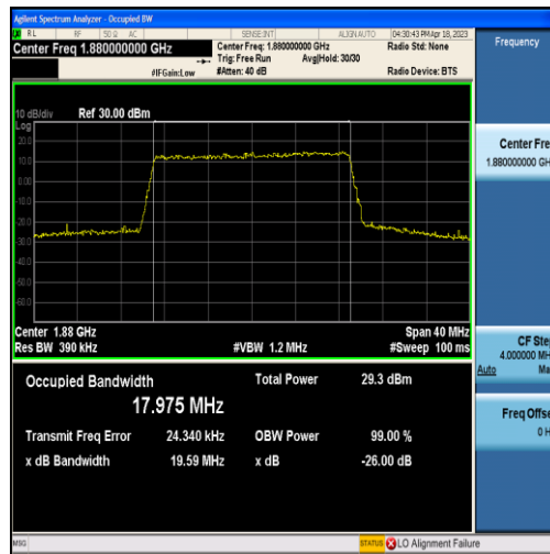
Band2-20MHz-QPSK-18900-100RB#0-17.975
