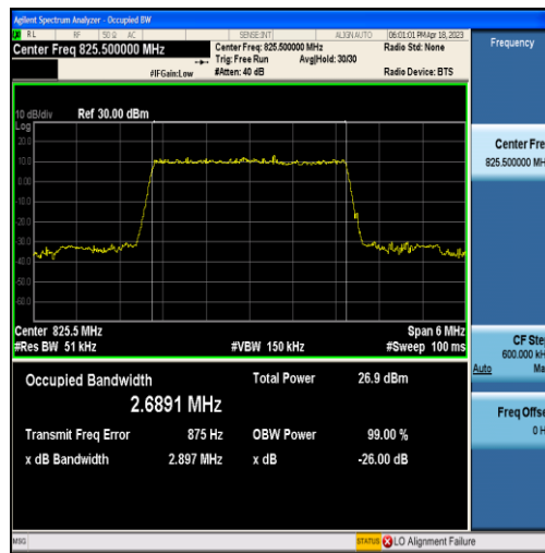
Band5-3MHz-QPSK-20415-15RB#0-2.6891
