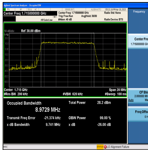
Band4-10MHz-QPSK-20000-50RB#0-8.9729
