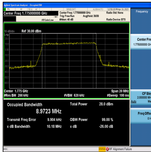
Band66-10MHz-QPSK-132622-50RB#0-8.9723
