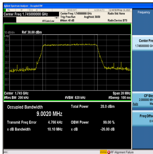
Band66-10MHz-QPSK-132322-50RB#0-9.0020
