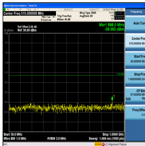
Band2-5MHz-QPSK-18900-25RB#0-Range1:30~1000MHz
