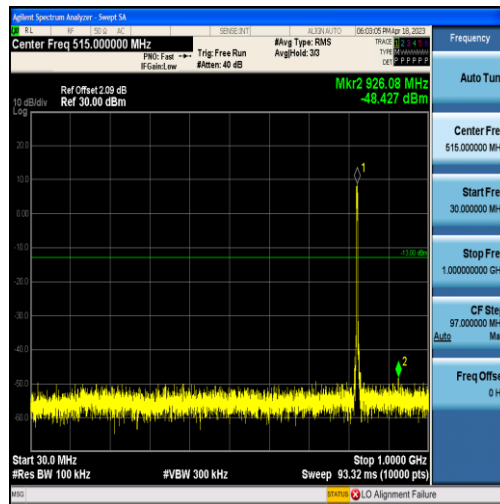
Band5-3MHz-QPSK-20415-15RB#0-Range1:30~1000MHz
