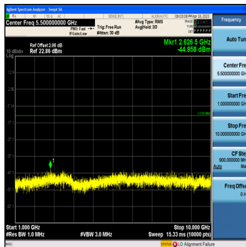
Band5-3MHz-QPSK-20415-15RB#0-Range2:1000~10000MHz
