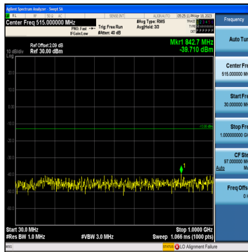
Band4-10MHz-QPSK-20350-50RB#0-Range1:30~1000MHz
