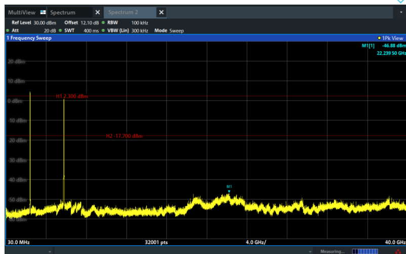
Antenna port: 1
