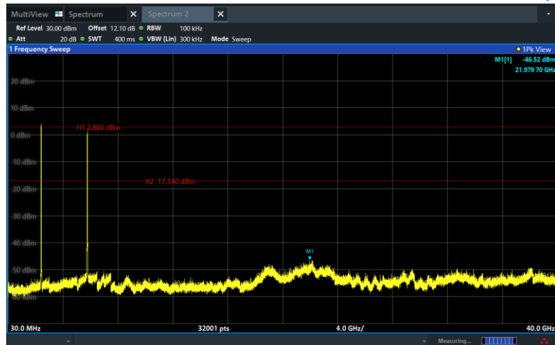
Antenna port: 1
