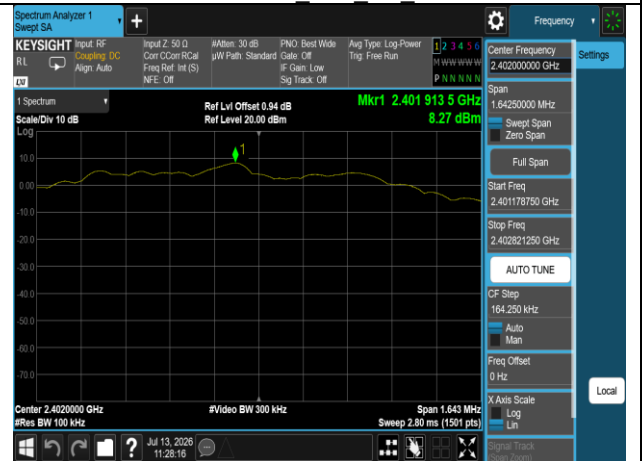
Reference Level BLE 2M 2402MHz
