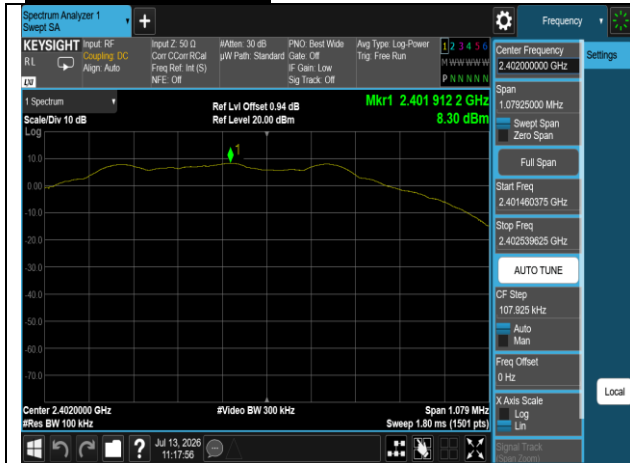
Reference Level BLE 1M 2402MHz
