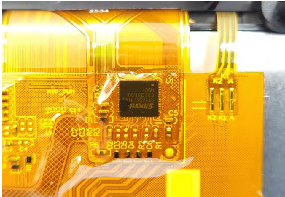
EUT Photo (53)
