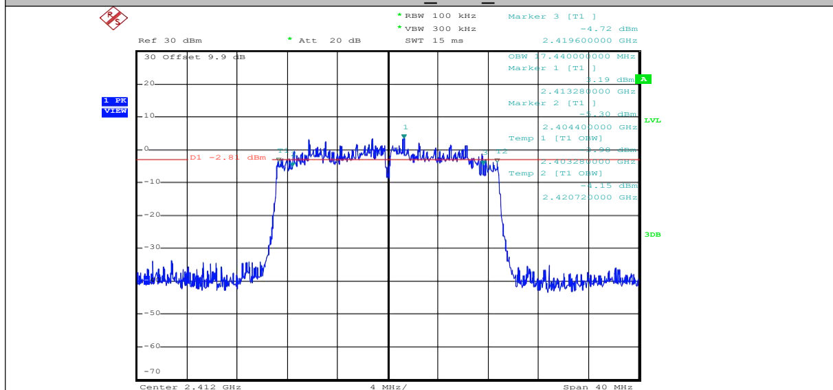
11N20MIMO_Ant0_2412
