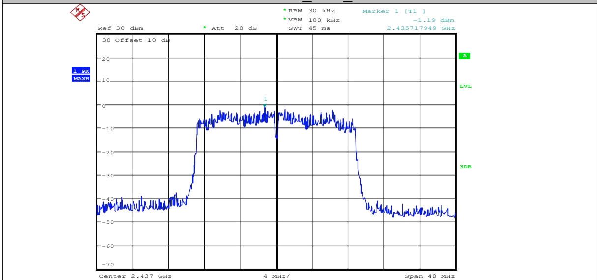
11N20MIMO_Ant1_2437
