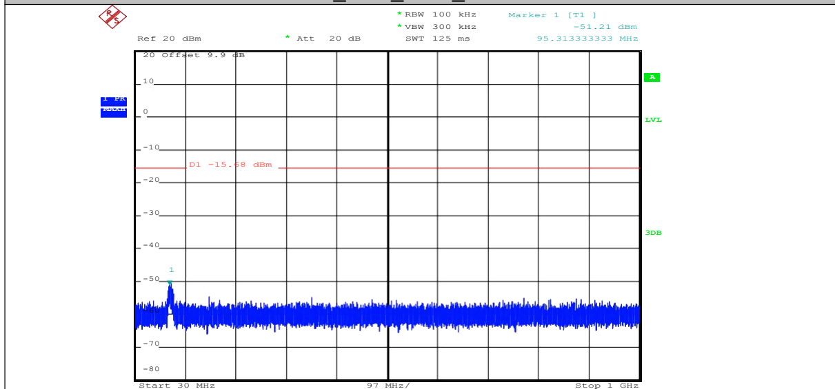
11G_Ant0_2412_30~1000
