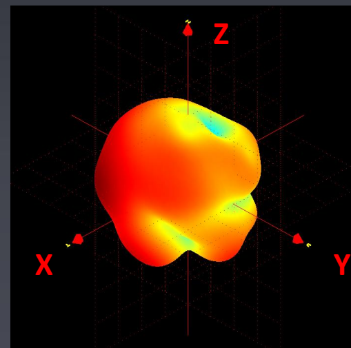
2440MHz 3D方向图
