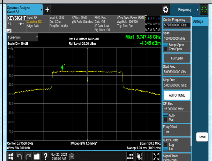
11AC80SISO-Ant1-5775-PASS
