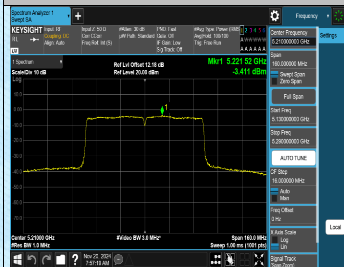
11AC80SISO-Ant1-5210-PASS
