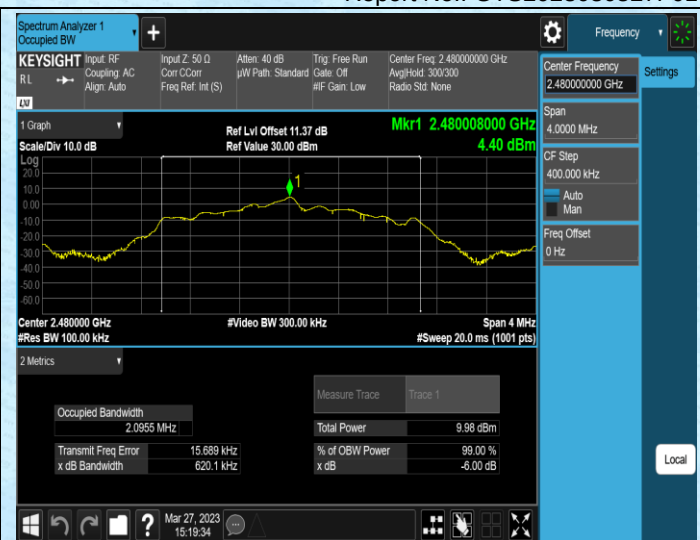
BLE_2M-Ant1-2480
