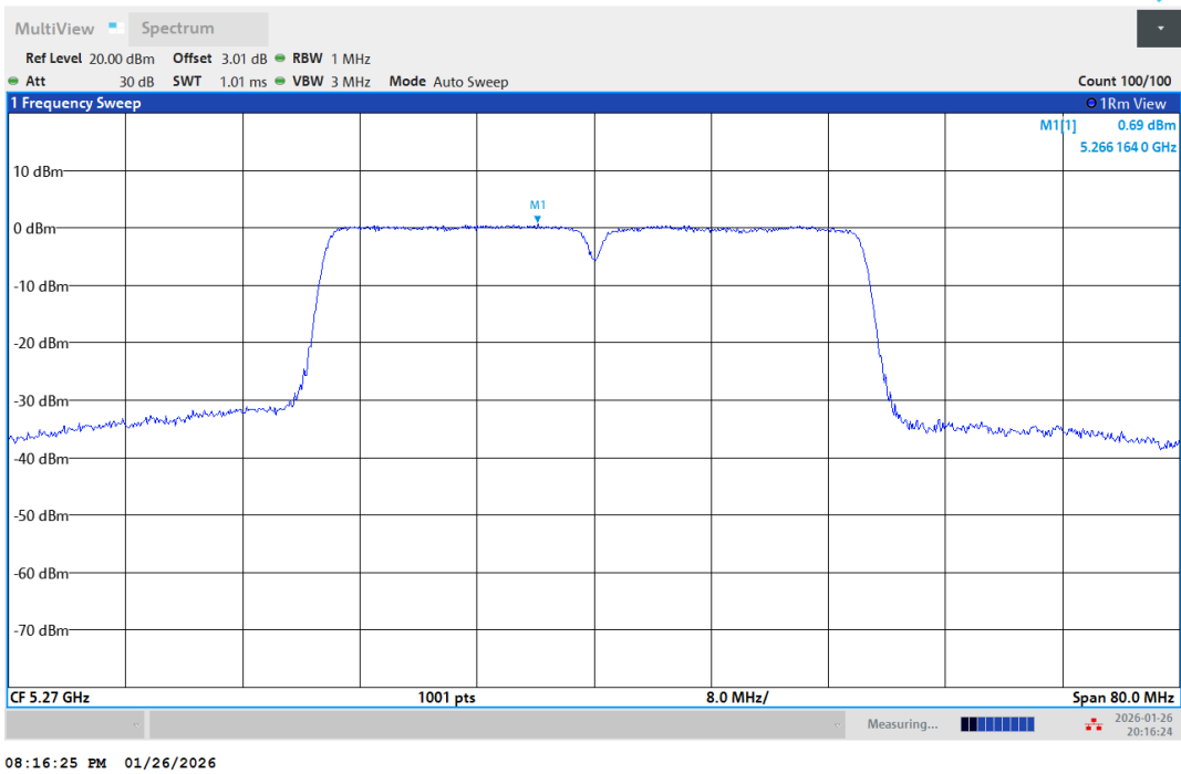
11AC40-5270-PASS
