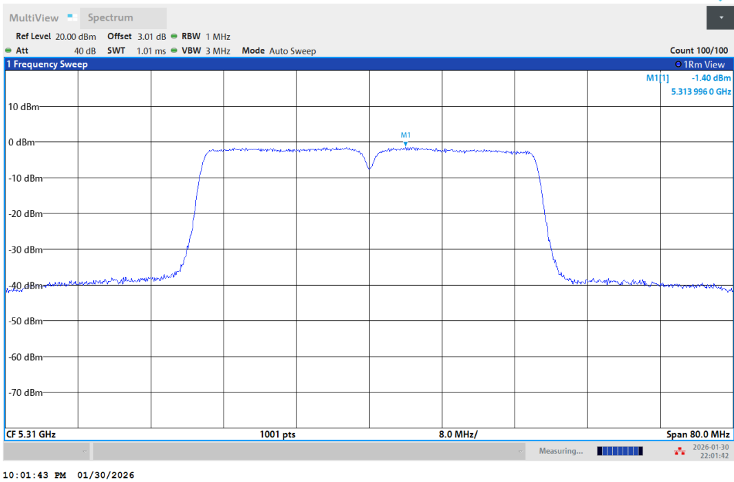
11AC40-5310-PASS
