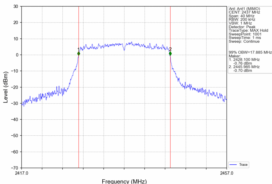
802.11n(HT20)_MCH_2437MHz_Ant1 (MIMO)_NTNV
