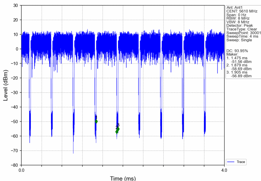
802.11ax(HEW80)_HCH_5610MHz_RU996_Left_Ant1_NTNV
