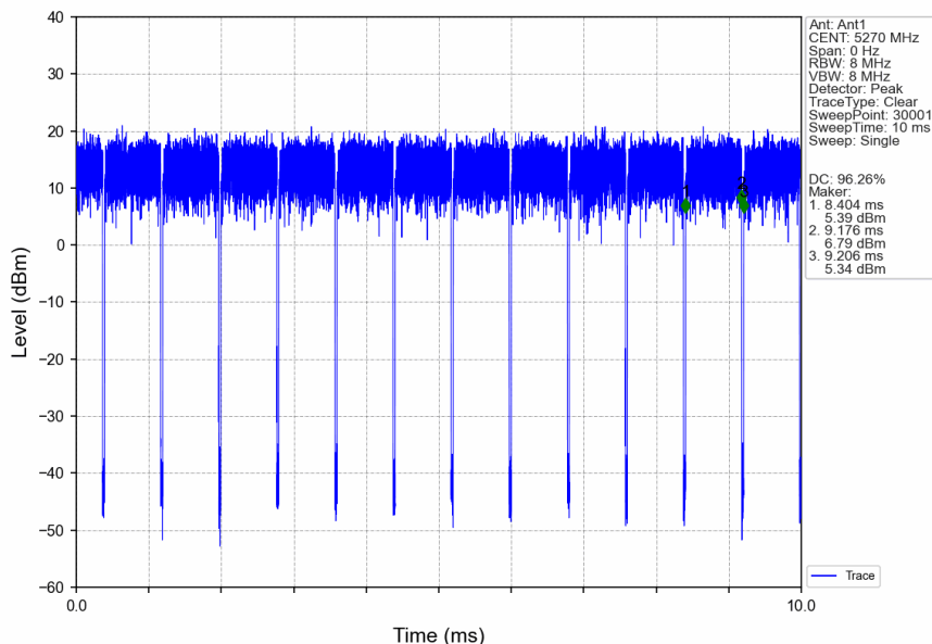
802.11ax(HEW40)_LCH_5270MHz_RU484_Left_Ant1_NTNV
