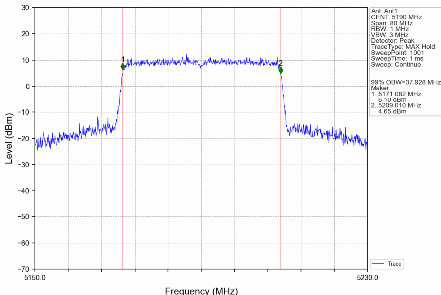
802.11ax(HEW40)_LCH_5190MHz_RU484_Left_Ant1_NTNV
