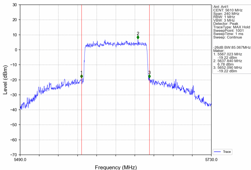
802.11ax(HEW80)_HCH_5610MHz_RU996_Left_Ant1_NTNV
