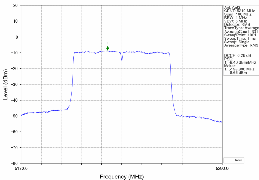
802.11ac(VHT80)_MCH_5210MHz_Ant2_NTNV
