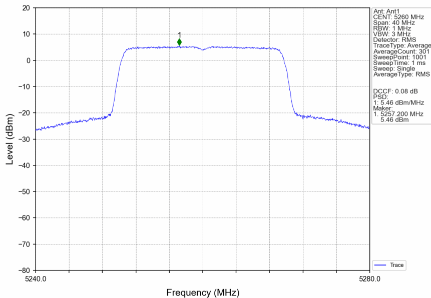
802.11ax(HEW20)_LCH_5260MHz_RU242_Left_Ant1_NTNV
