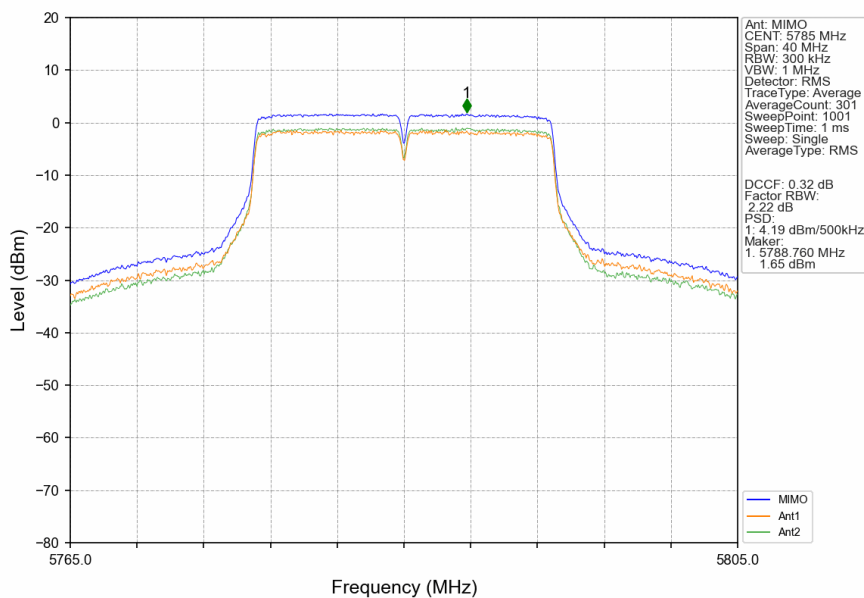
802.11n(HT20)_MCH_5785MHz_MIMO_NTNV
