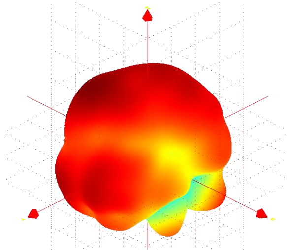
5190MHz 3D
