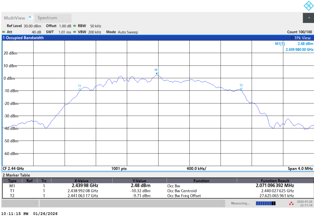
BLE_2M-Ant1-2440
