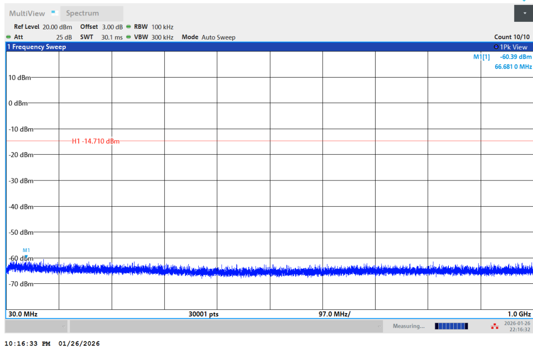
BLE_2M-Ant1-2440-30~1000-PASS
