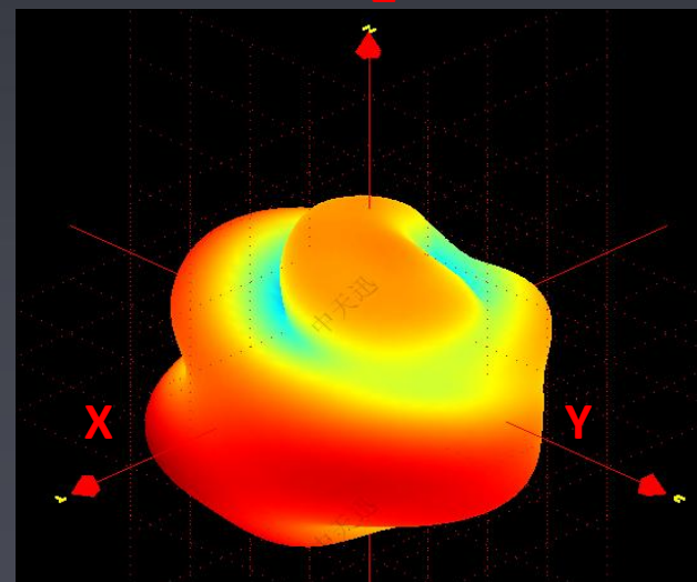
2450MHz 3D方向图
