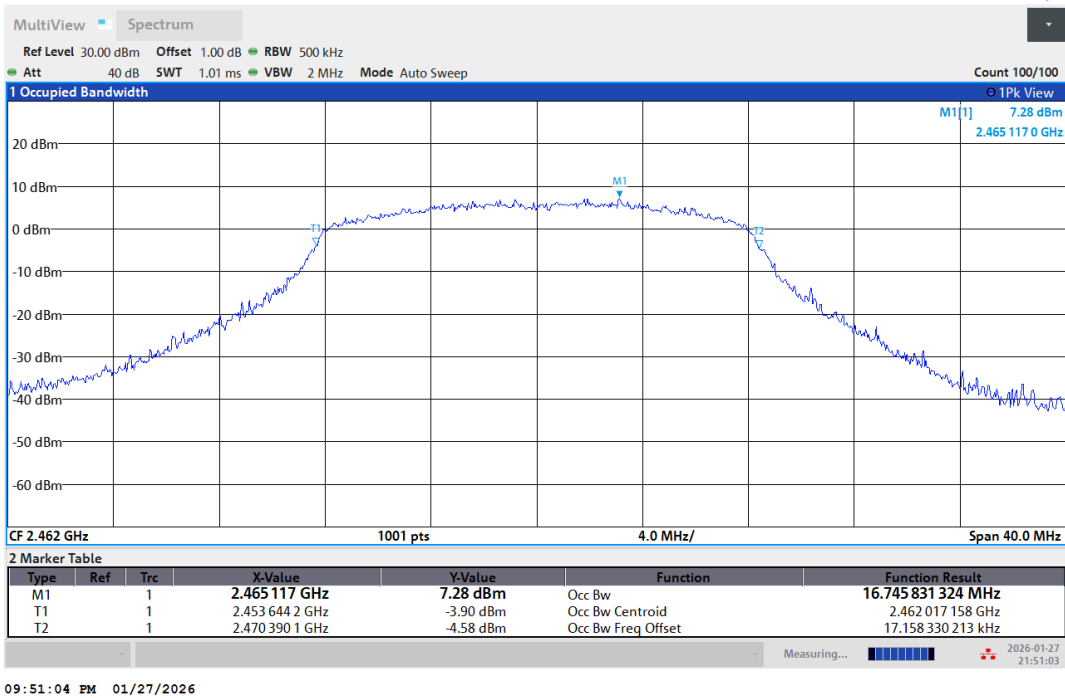
11G-Ant1-2462
