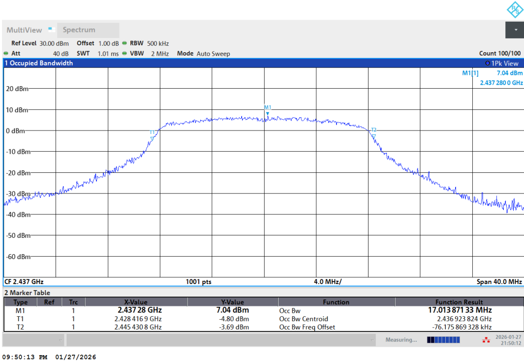
11G-Ant1-2437
