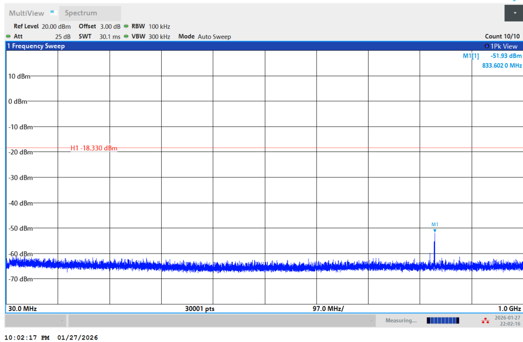
11G-Ant1-2437-30~1000-PASS
