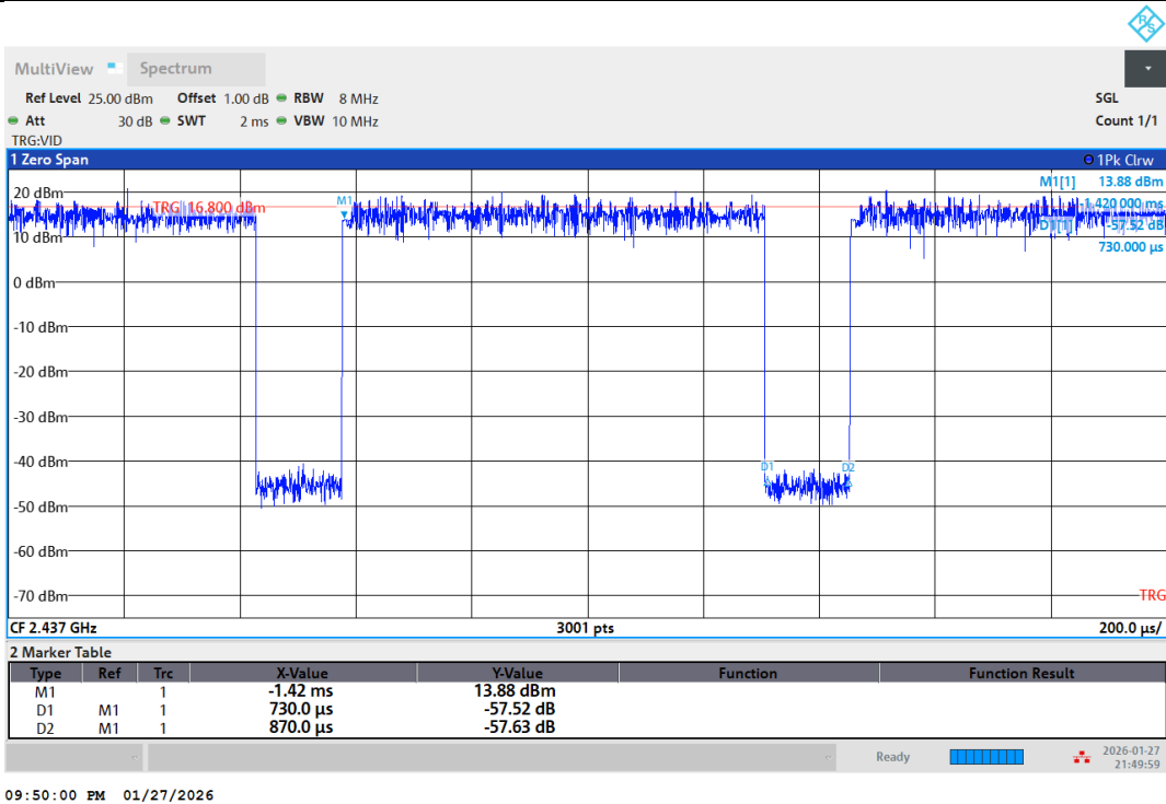
NTNV-11G-Ant1-2437
