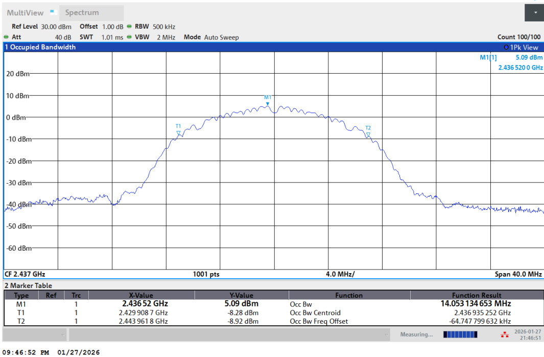
11B-Ant1-2437
