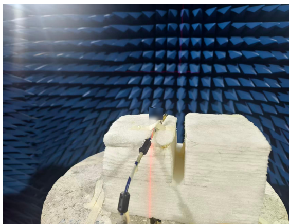
YOZ面 ( \phi=90^\circ )
