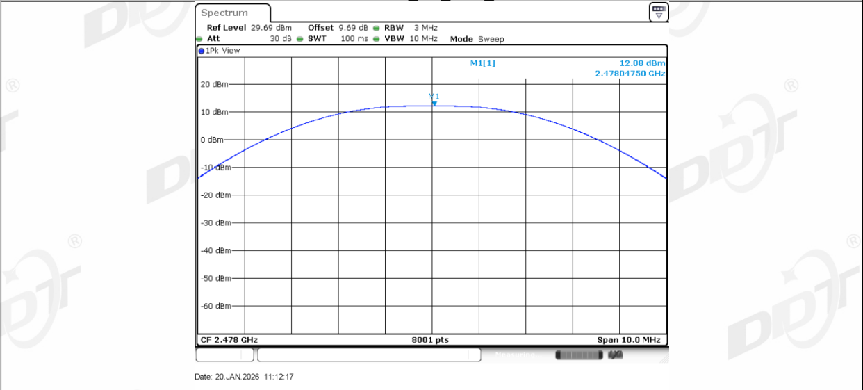
2.4G SRD_2M_Ant2_2478
