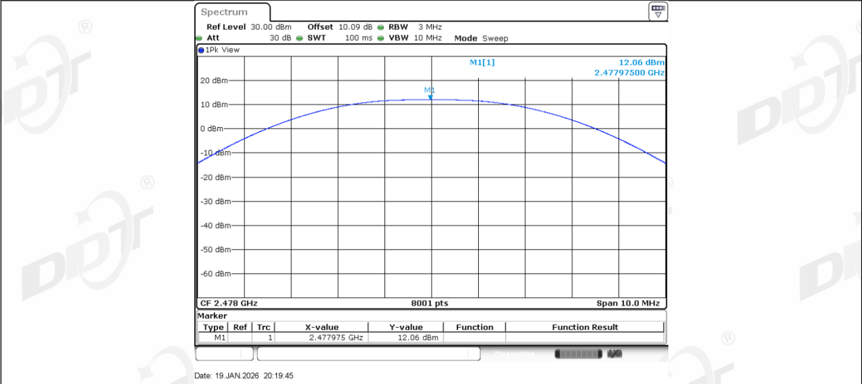
2.4G SRD_2M_Ant2_2478
