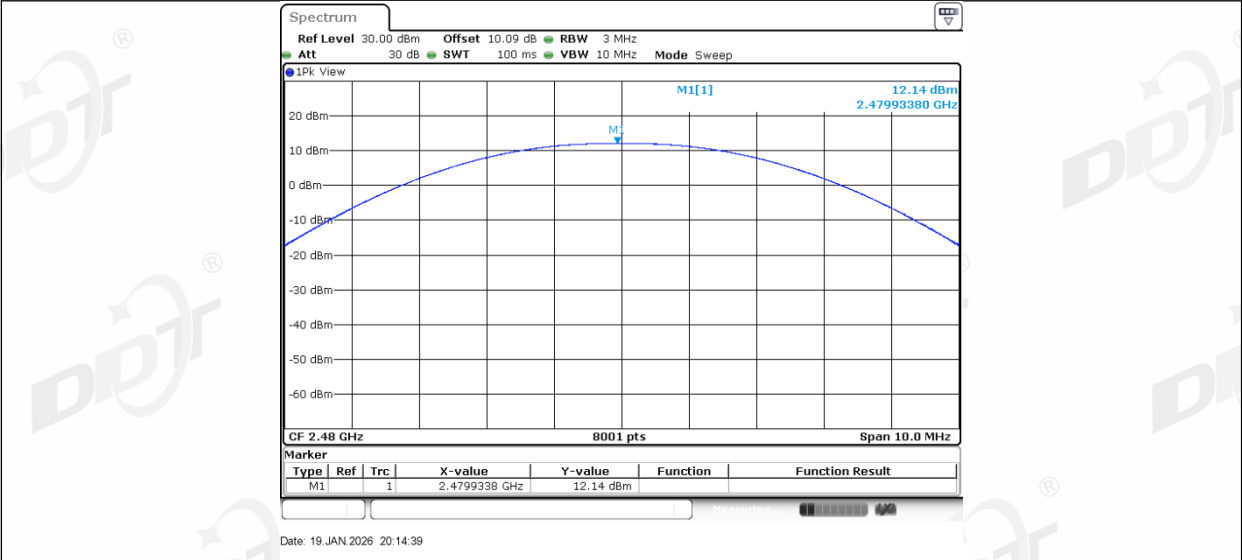
2.4G SRD_1M_Ant2_2480
