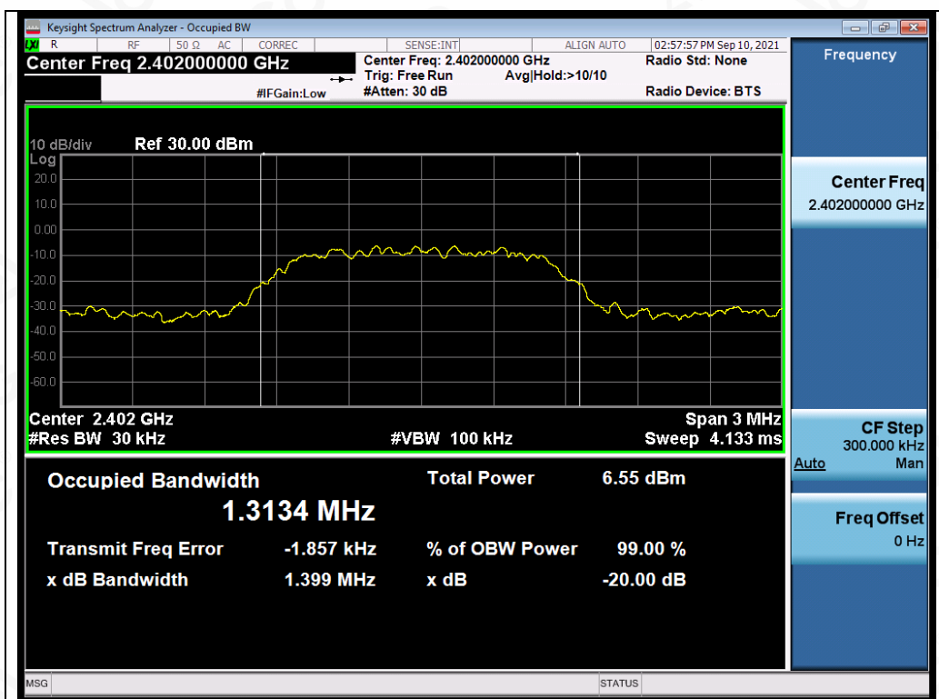
Test_Graph_EDR_ANT1_2402_2Mbps_OBW
