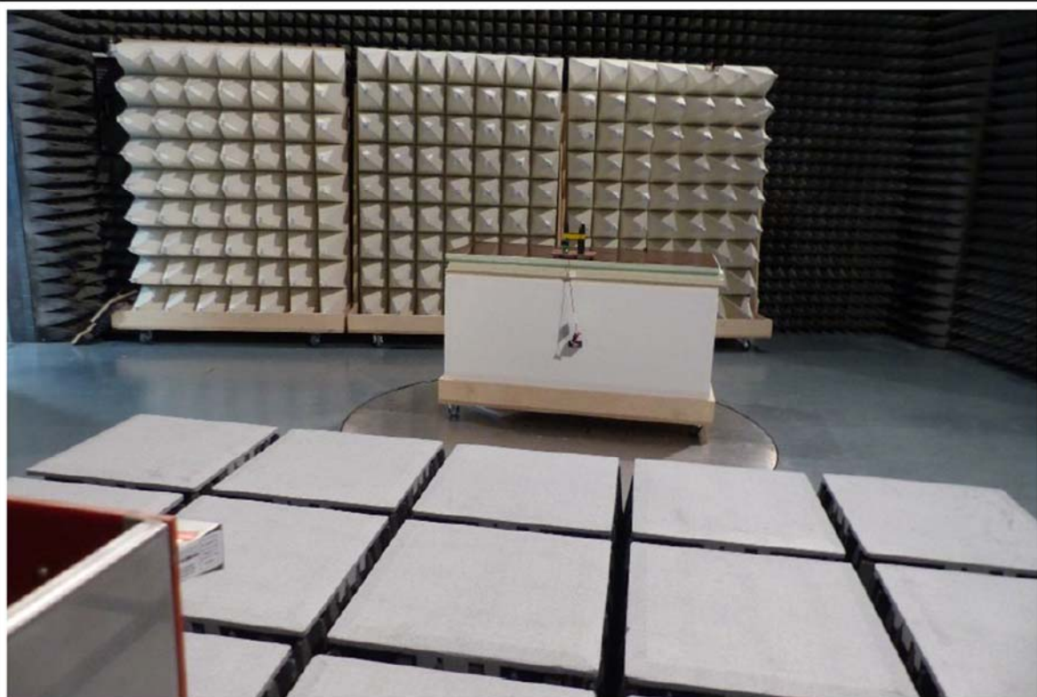
Test setup BLE 17-26.5GHz
