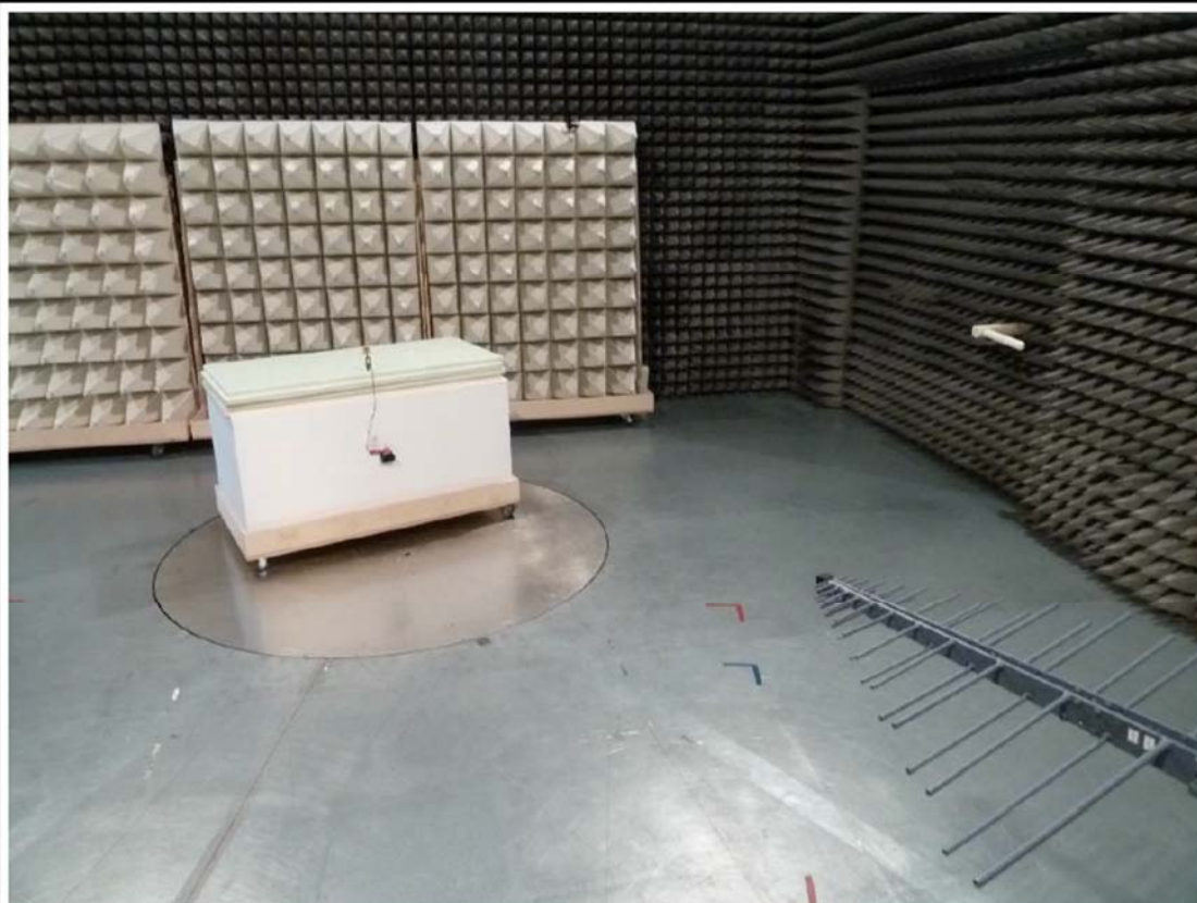
Test setup UWB 200-1000MHz
