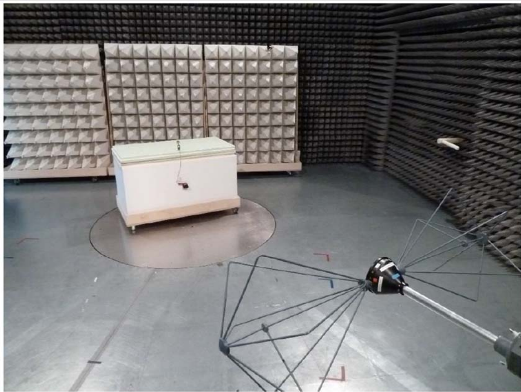
Test setup UWB 30-200MHz
