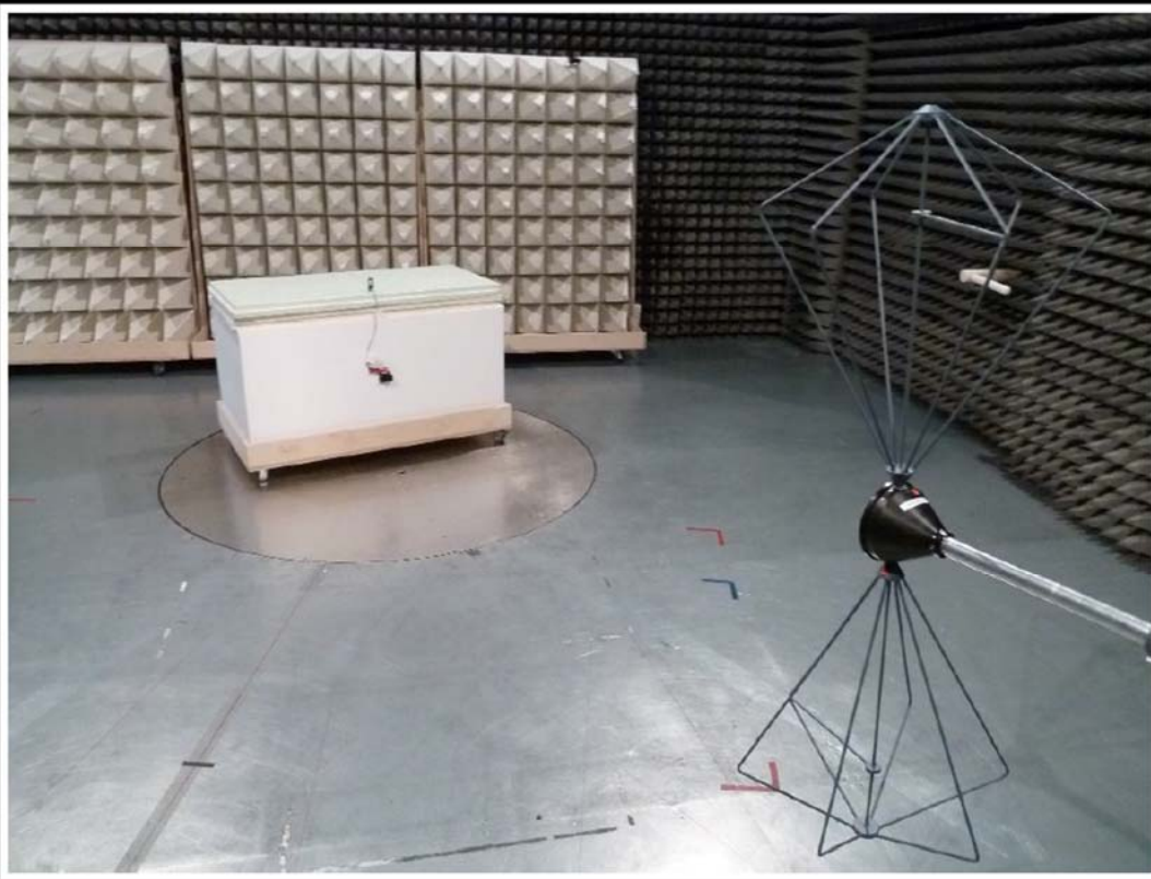
Test setup BLE 30-200MHz
