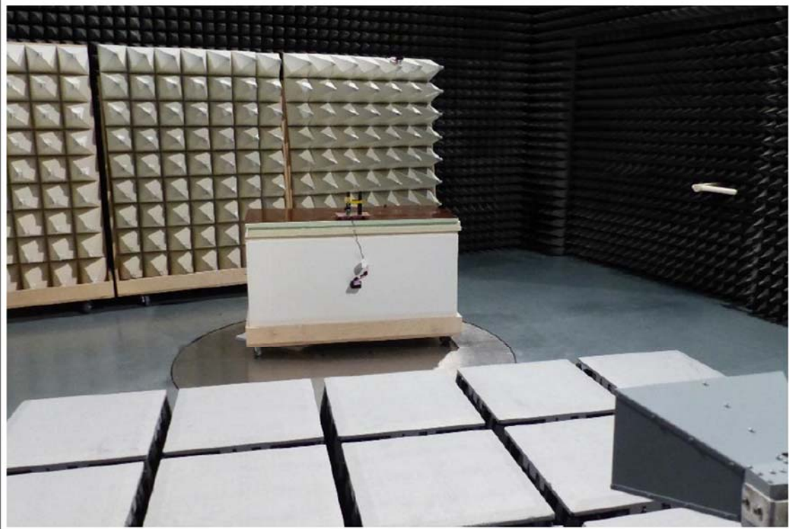
Test setup UWB 1-17GHz
