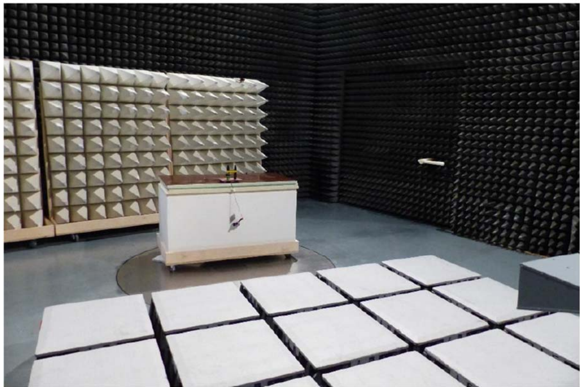
Test setup BLE 1-17GHz
