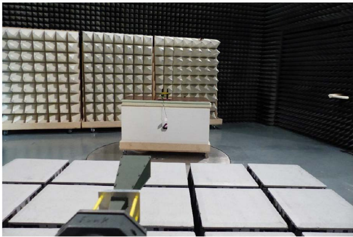
Test setup BLE 26.5-40GHz
