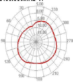
2450.000MHz H
