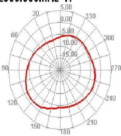
2500.000MHz H
