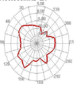
2400.000MHz E1
