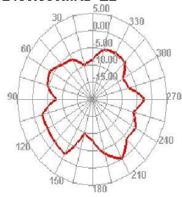
2400.000MHz E2
