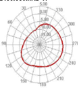
2400.000MHz H
