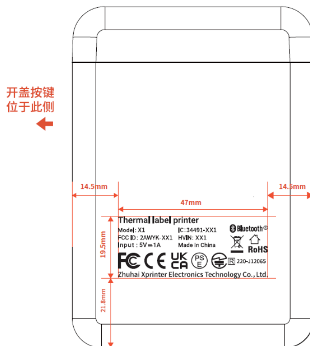
该镭雕位于打印机背面
