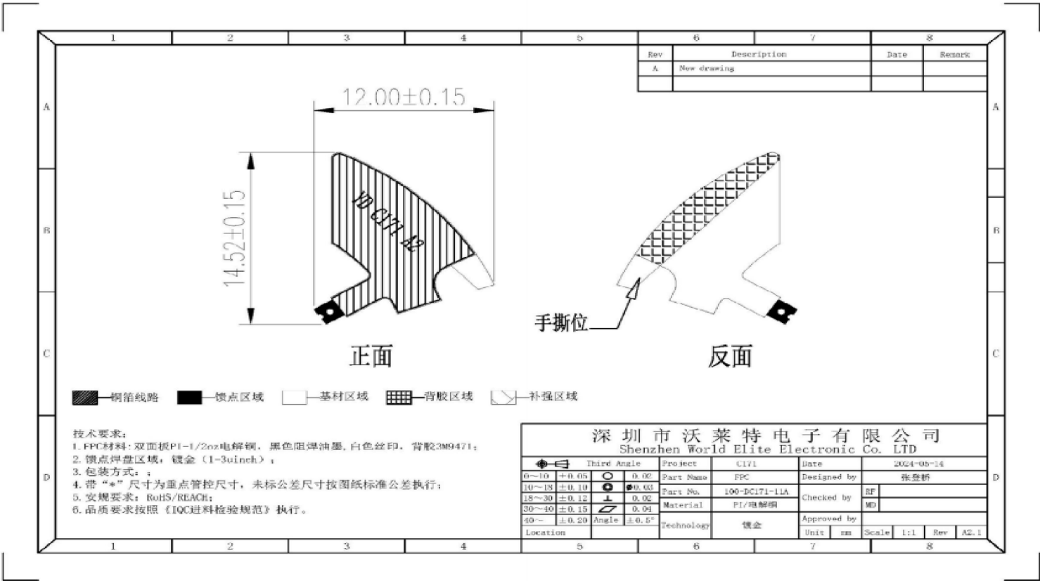
图2 产品结构图
