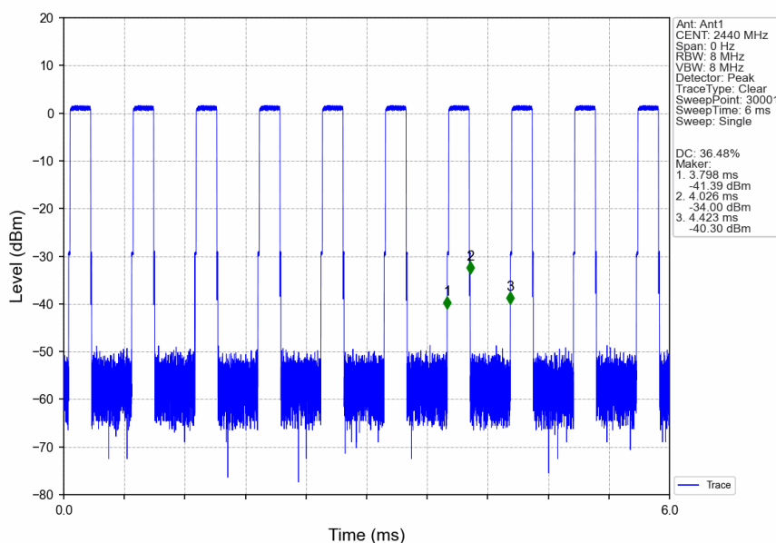
2M_MCH_2440MHz_Ant1_NTNV
