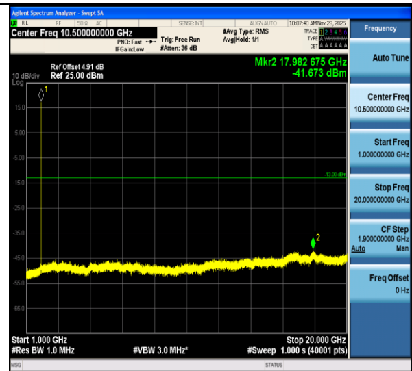
Band II-9400-1000~20000MHz-PASS
