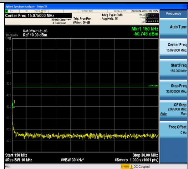
Band II-9538-0.15~30MHz-PASS
