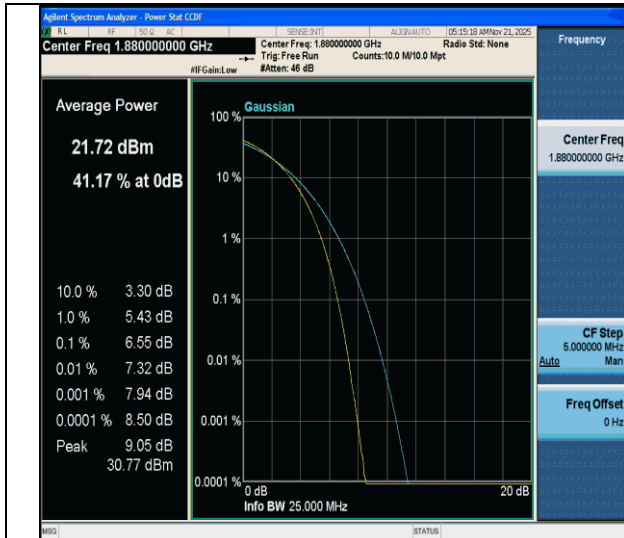
CA_2C-20MHz-20MHz-QPSK-QPSK-18801-18999-100RB#0-100RB#0-PASS
