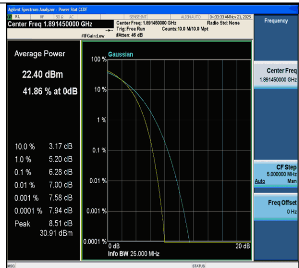
CA_2C-15MHz-20MHz-QPSK-QPSK-18929-19100-75RB#0-100RB#0-PASS
