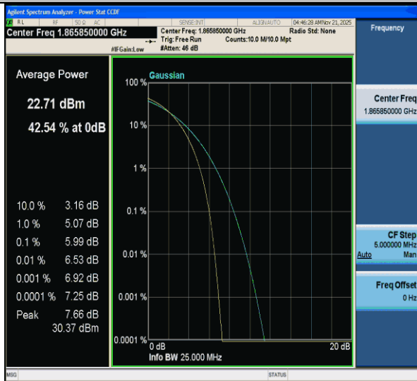
CA_2C-20MHz-5MHz-QPSK-QPSK-18700-18817-100RB#0-25RB#0-PASS
