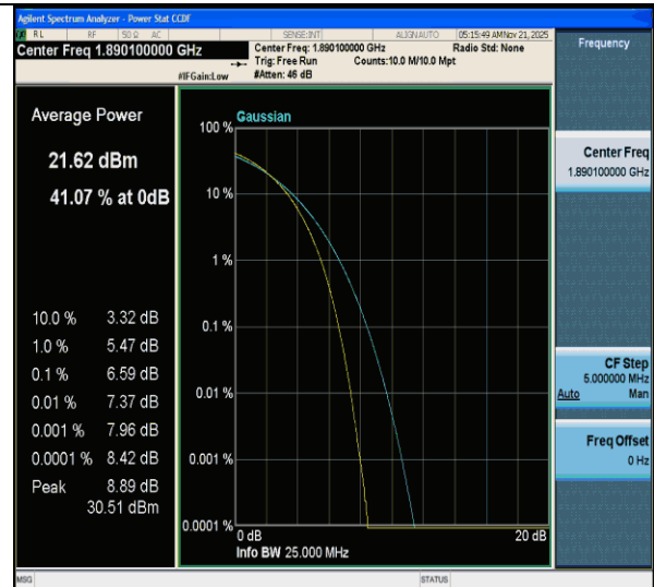
CA_2C-20MHz-20MHz-QPSK-QPSK-18902-19100-100RB#0-100RB#0-PASS
