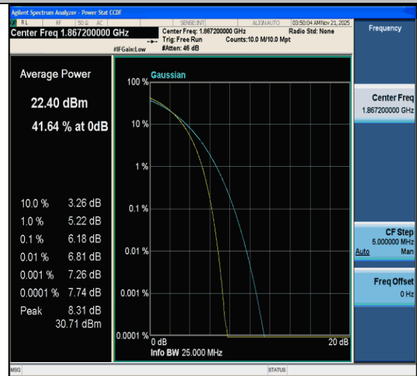
CA_2C-20MHz-10MHz-QPSK-QPSK-18700-18844-100RB#0-50RB#0-PASS
