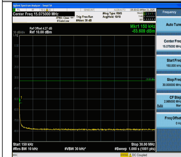
CA_2C-20MHz-20MHz-QPSK-QPSK-18801-18999-1RB#0- ORB#0-0.15~30MHz-PASS
