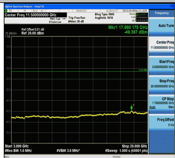
CA_2C-20MHz-20MHz-QPSK-QPSK-18801-18999-1RB#0- ORB#0-3000~20000MHz-PASS
