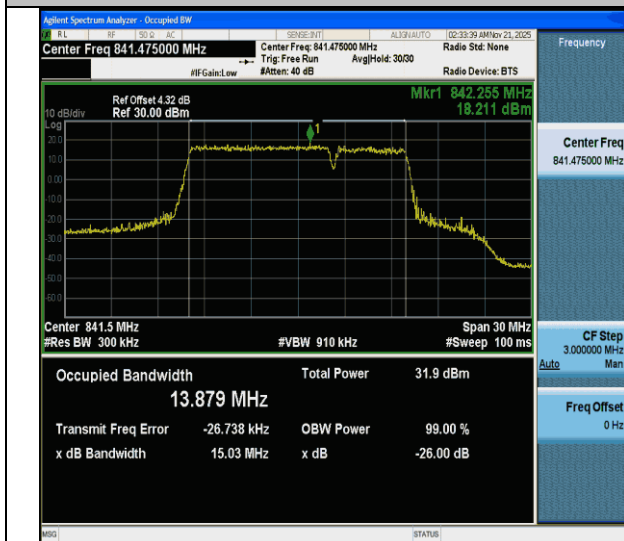
CA_5B-10MHz-5MHz-QPSK-QPSK-20550-20622-50RB#0-25RB#0-PASS
