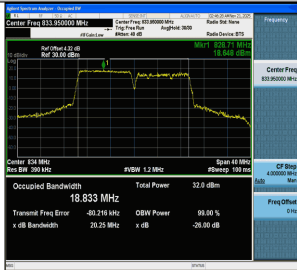
CA_5B-10MHz-10MHz-QPSK-QPSK-20450-20549-50RB#0- 50RB#0-PASS
