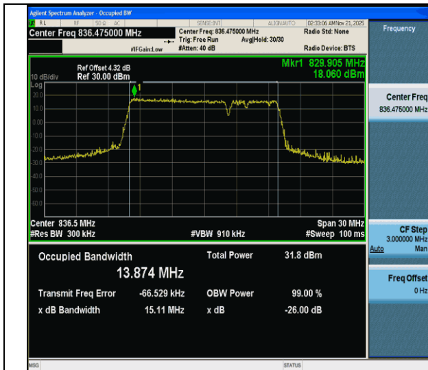
CA_5B-10MHz-5MHz-QPSK-QPSK-20500-20572-50RB#0-25RB#0-PASS
