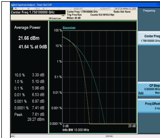
CA_66B-10MHz-5MHz-QPSK-QPSK-132397-132469-50RB#0-25RB#0-PASS
