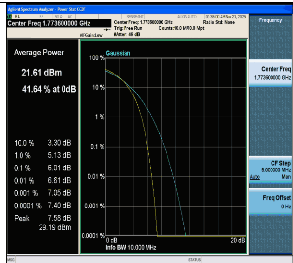
CA_66B-10MHz-5MHz-QPSK-QPSK-132572-132644-50RB#0-25RB#0-PASS
