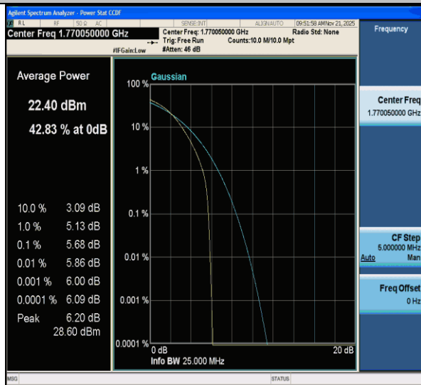
CA_66B-10MHz-10MHz-QPSK-QPSK-132523-132622-50RB#0-50RB#0-PASS
