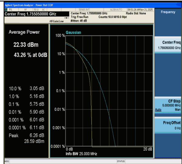
CA_66B-10MHz-10MHz-QPSK-QPSK-132373-132472-50RB#0-50RB#0-PASS
