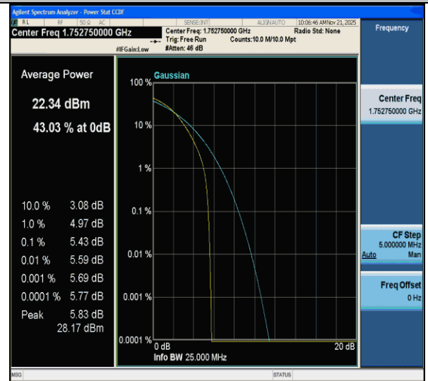
CA_66B-5MHz-15MHz-QPSK-QPSK-132353-132446-25RB#0-75RB#0-PASS
