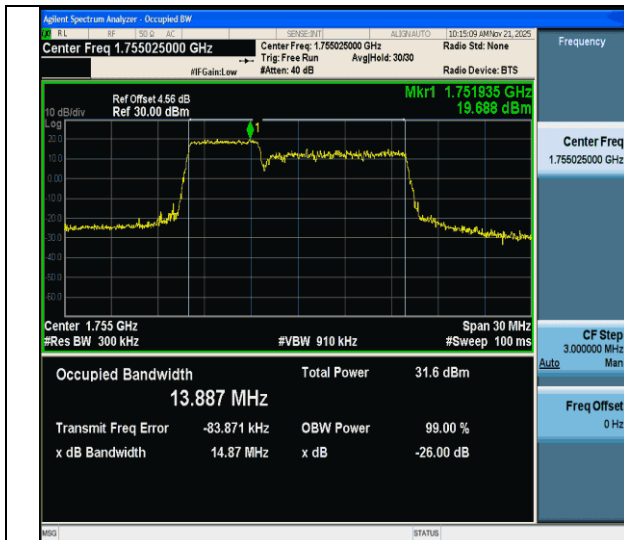
CA_66B-5MHz-10MHz-QPSK-QPSK-132375-132447-25RB#0-50RB#0-PASS
